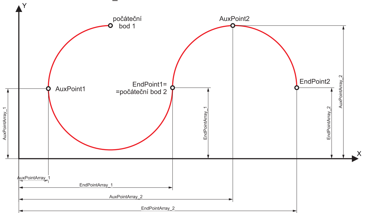
MC_MoveCircularAbsolute - Příklad
