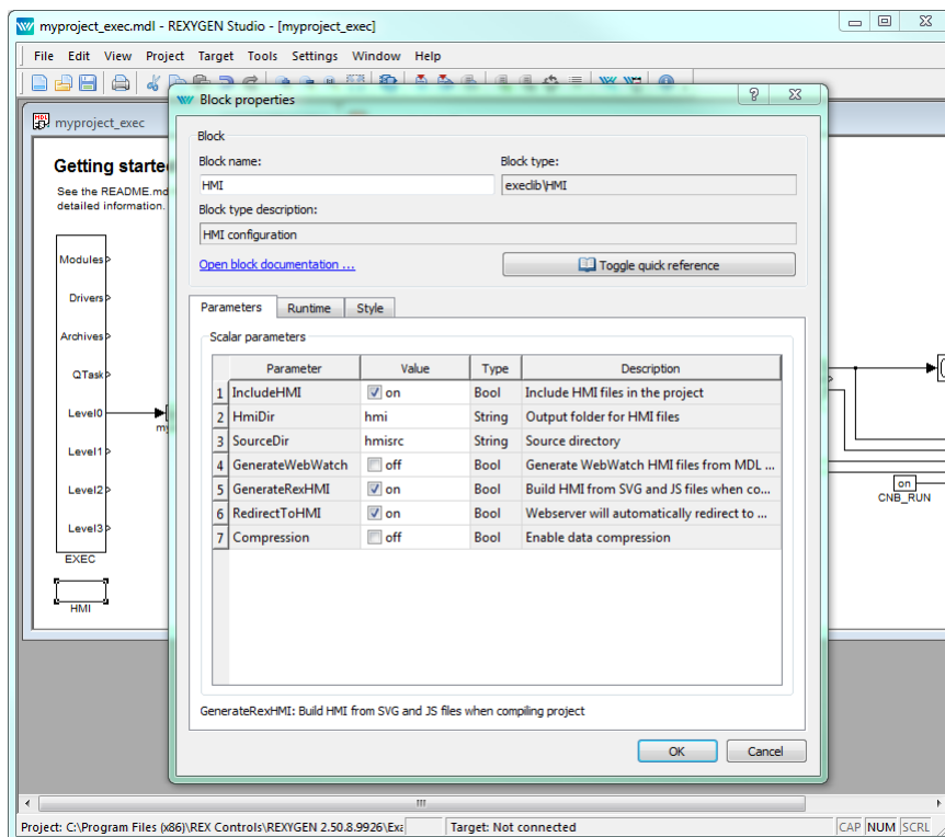
Obrázek 1.2: Konfigurace bloku HMI v REXYGEN Studio
